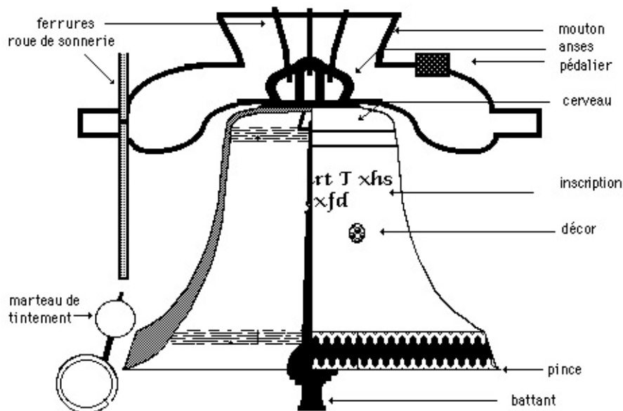
Shéma d'une cloche extrait du vocabulaire campanaire de la société française campanaire © campanologie.free.fr
